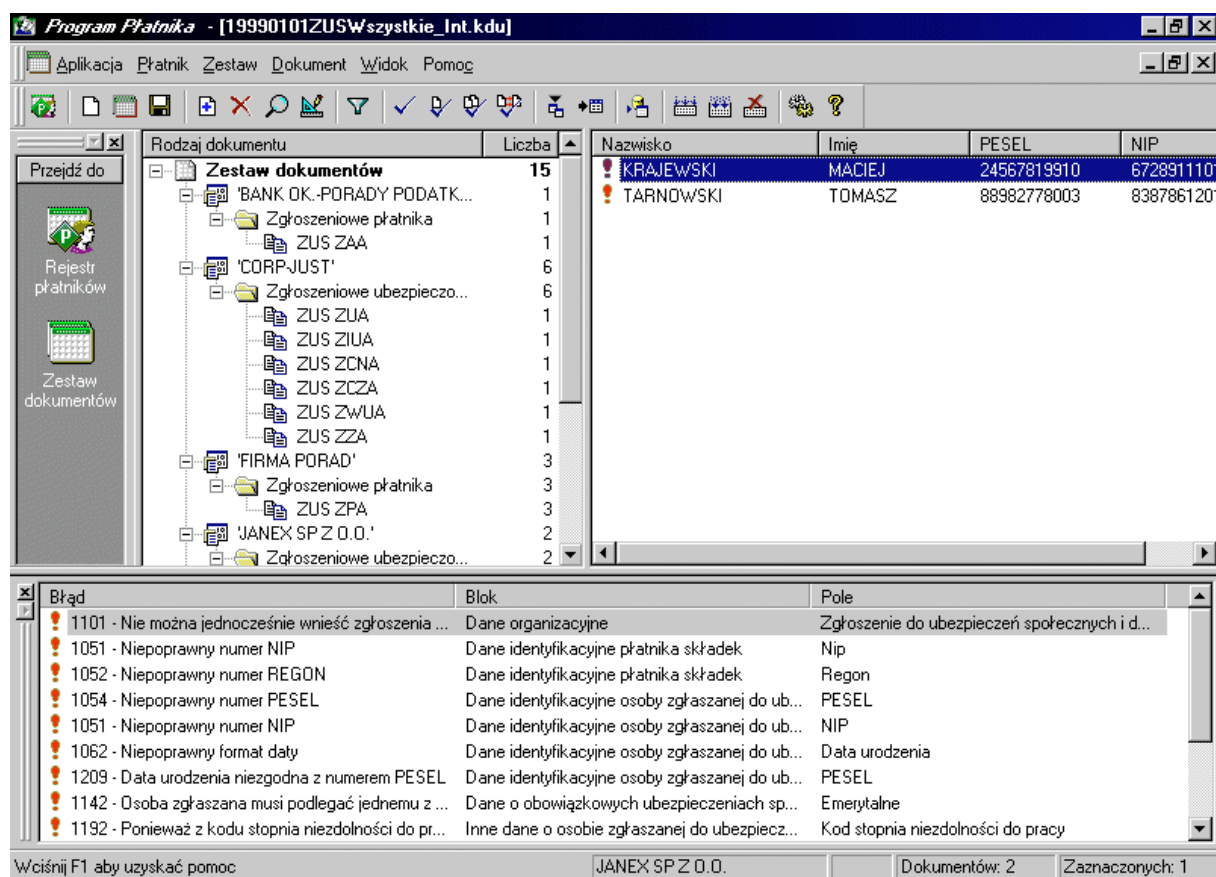
Rysunek 60. Okno robocze - weryfikacja dokumentu
