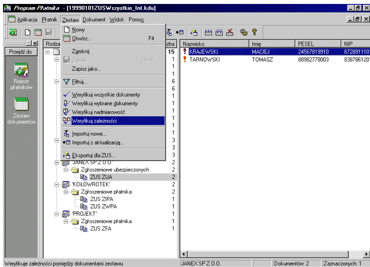
Rysunek 47. Okno robocze - weryfikacja zależności między dokumentami w zestawie
