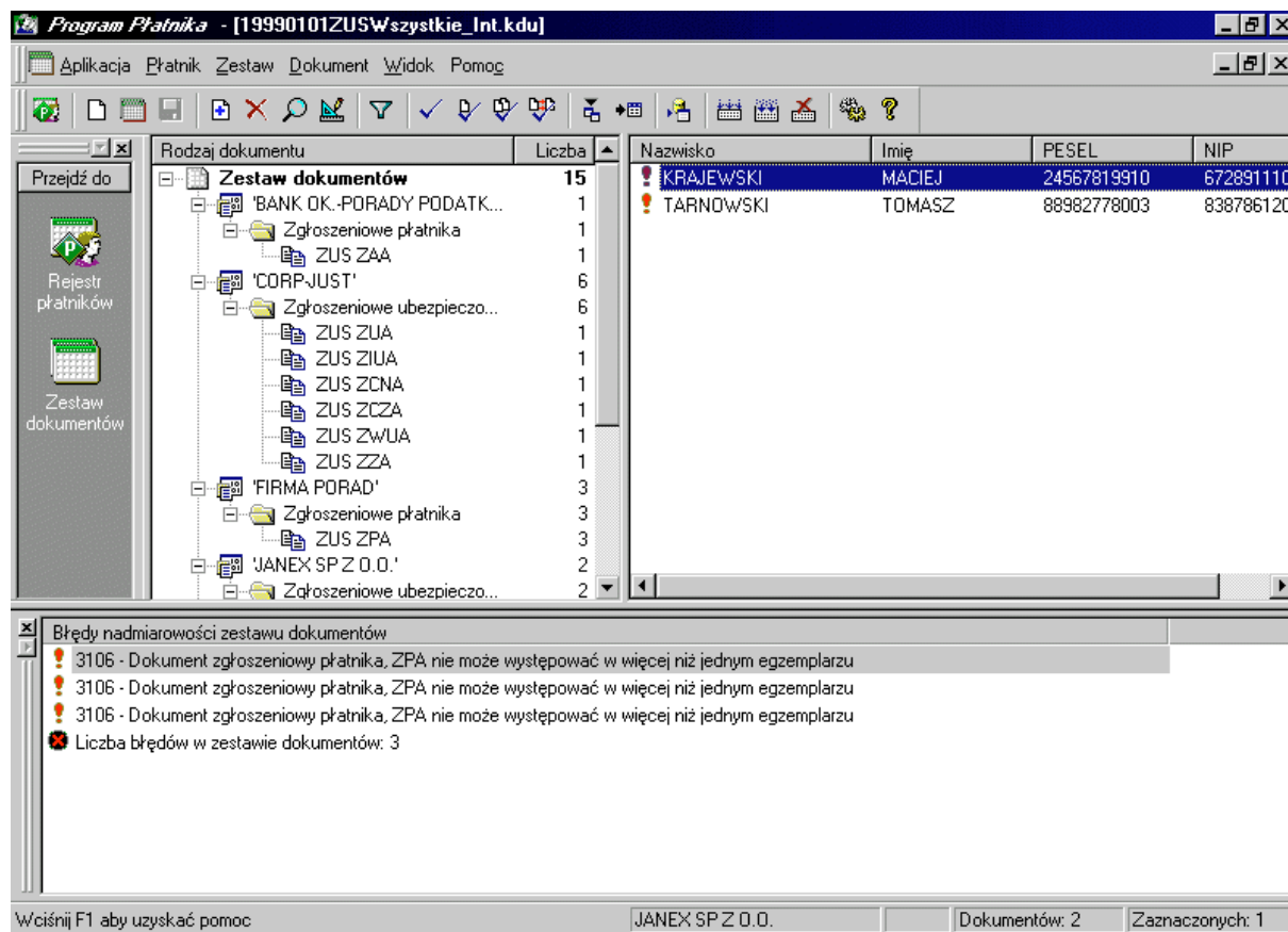
Rysunek 46. Okno robocze – raport z weryfikacji nadmiarowości dokumentów w zestawie
